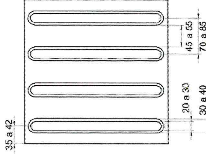
Signalização tátil direcional – Modulação do piso (dimensões em mm)
