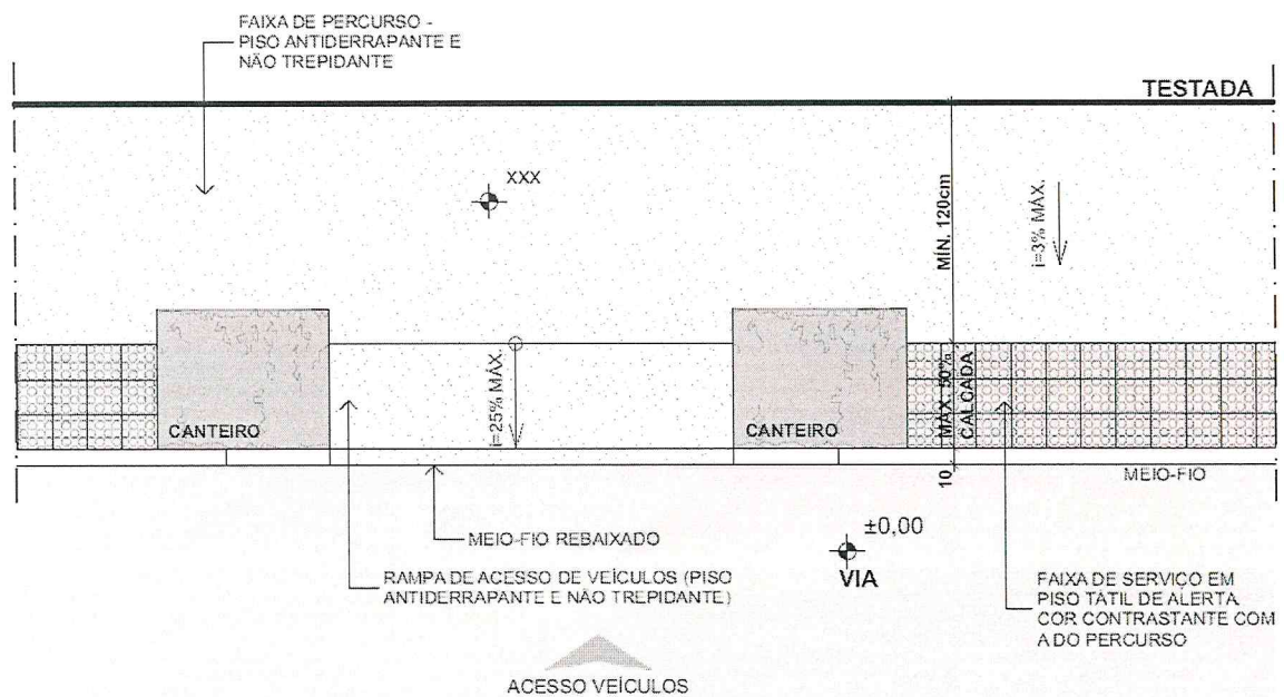
Figura 3 - Rebaixamento de meio-fio entre canteiros
