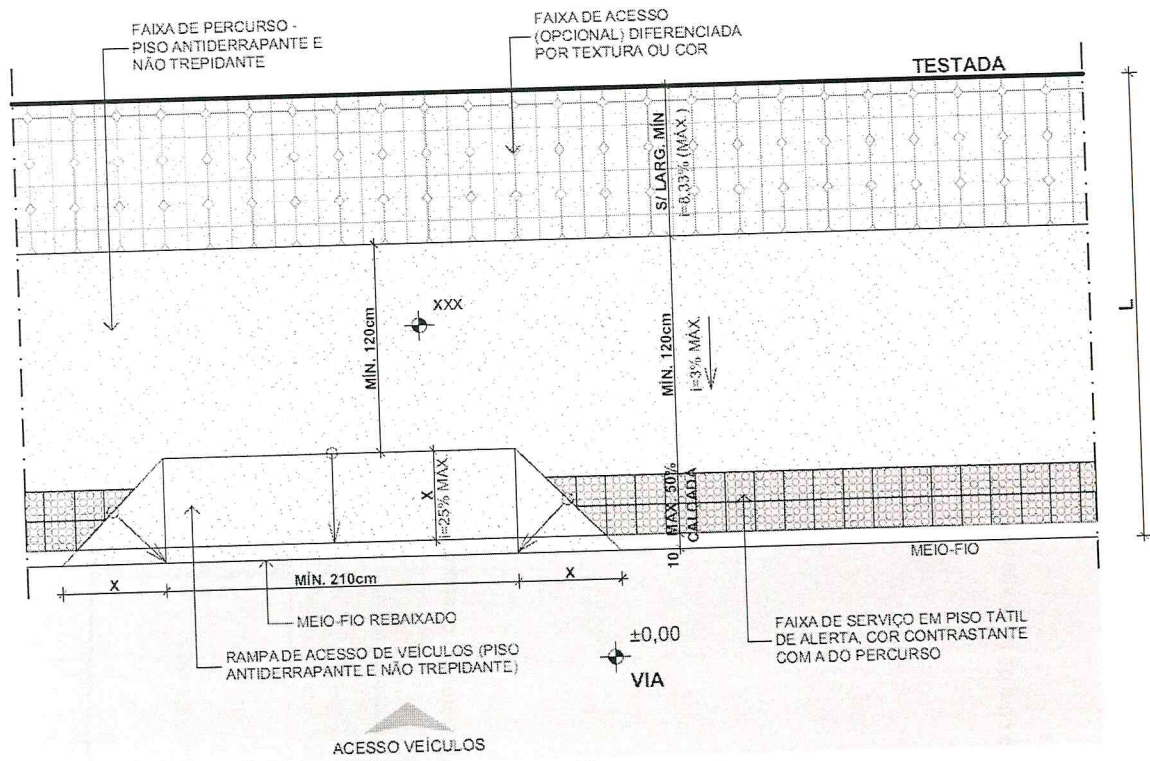
Figura 4 - Calçada com 03 faixas diferenciadas - L > 2,00m
